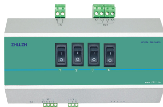
图 1：4 路高可靠调光模块
